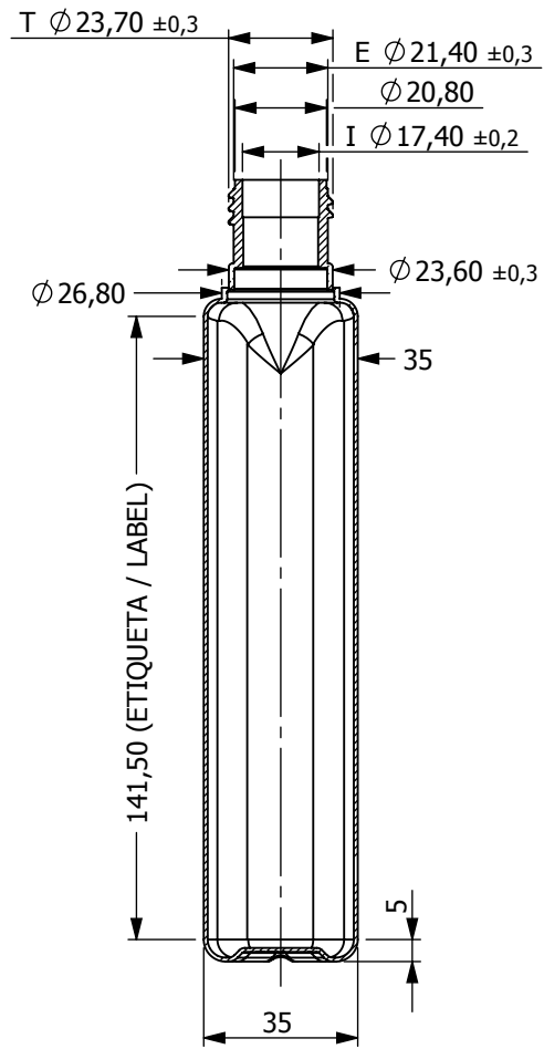
SECCIÓN/SECTION A-A ESCALA/SCALE 1 : 1.9
