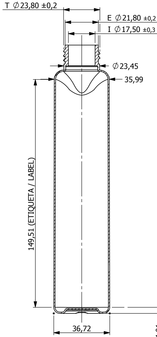
SECCIÓN/SECTION A-A ESCALA / SCALE 1 : 1.5
